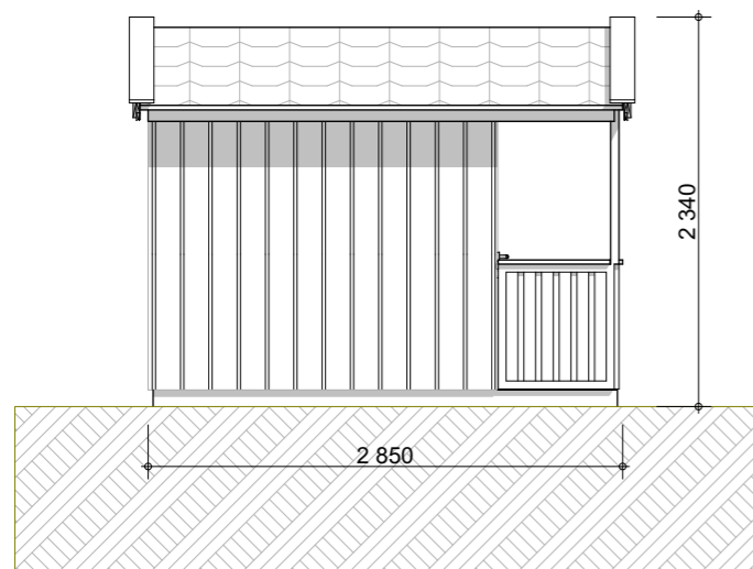
Fasade 1:50
