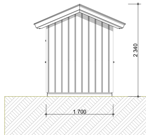
Fasade 1:50
