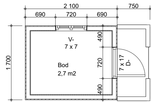
Plan 1:50
