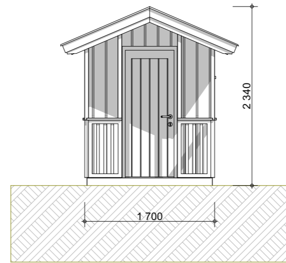
Fasade 1:50
