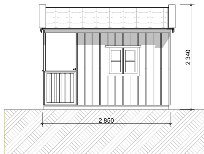
Fasade 1:50
